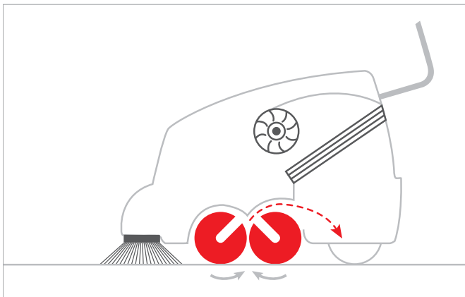
Das „TWS“-Prinzip The „TRS“-principle
